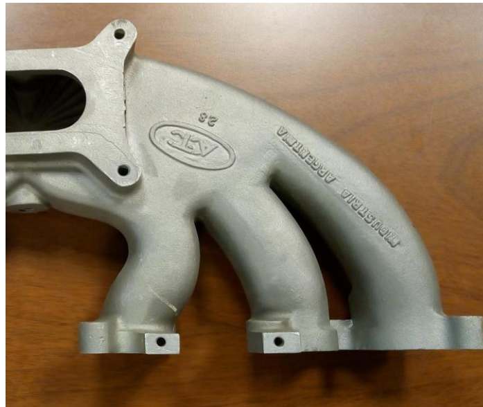
Figura 38.1 a - Múltiple Ford - Forma original de los tabiques
